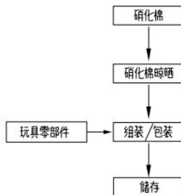
玩具类（玩具造型/桌面烟花）生产工艺流程图
